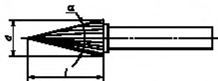
Рисунок 10 — Борфрезы типа М
