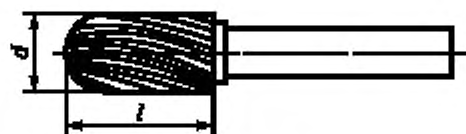
Рисунок 2 — Борфрезы типа С
