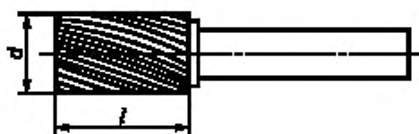
Рисунок 1 — Борфрезы типа А
