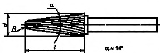
Рисунок 9 — Борфрезы типа L
