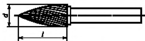
Рисунок 6 — Борфрезы типа G
