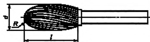
Рисунок 4 — Борфрезы типа E
