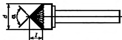
Рисунок 8 — Борфрезы типа J и K
